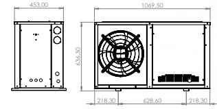
Karbox 2 Kabin
