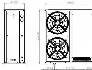
Karbox 10 Kabin
