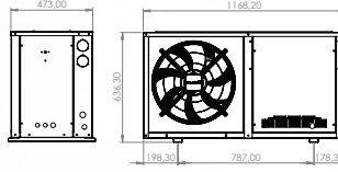
Karbox 3 Kabin
