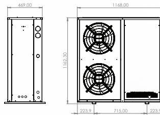
Karbox 5 Kabin
