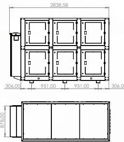
2500x1100 Kapalı Şase
