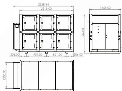
2500x1450 Kapalı Şase
