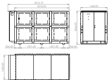
3000x1450 Kapalı Şase
