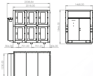
2000x1450 Kapalı Şase
