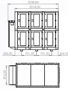
2000x1100 Kapalı Şase
