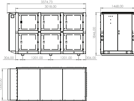
3000x1450 Kapalı Şase
